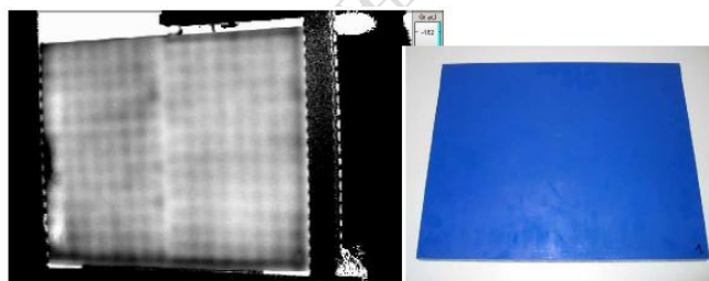
图 3：主动热成像法检测汽车仪表盘中的气孔
